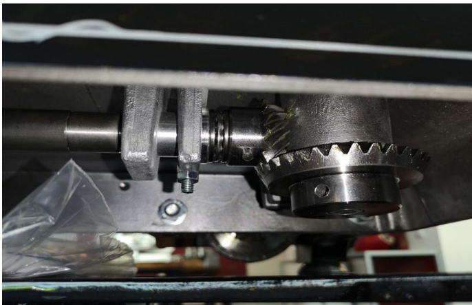
Zu fettende Zahnräder unter einer Volano – gültig für alle Volano (Schwungrad) Typen
